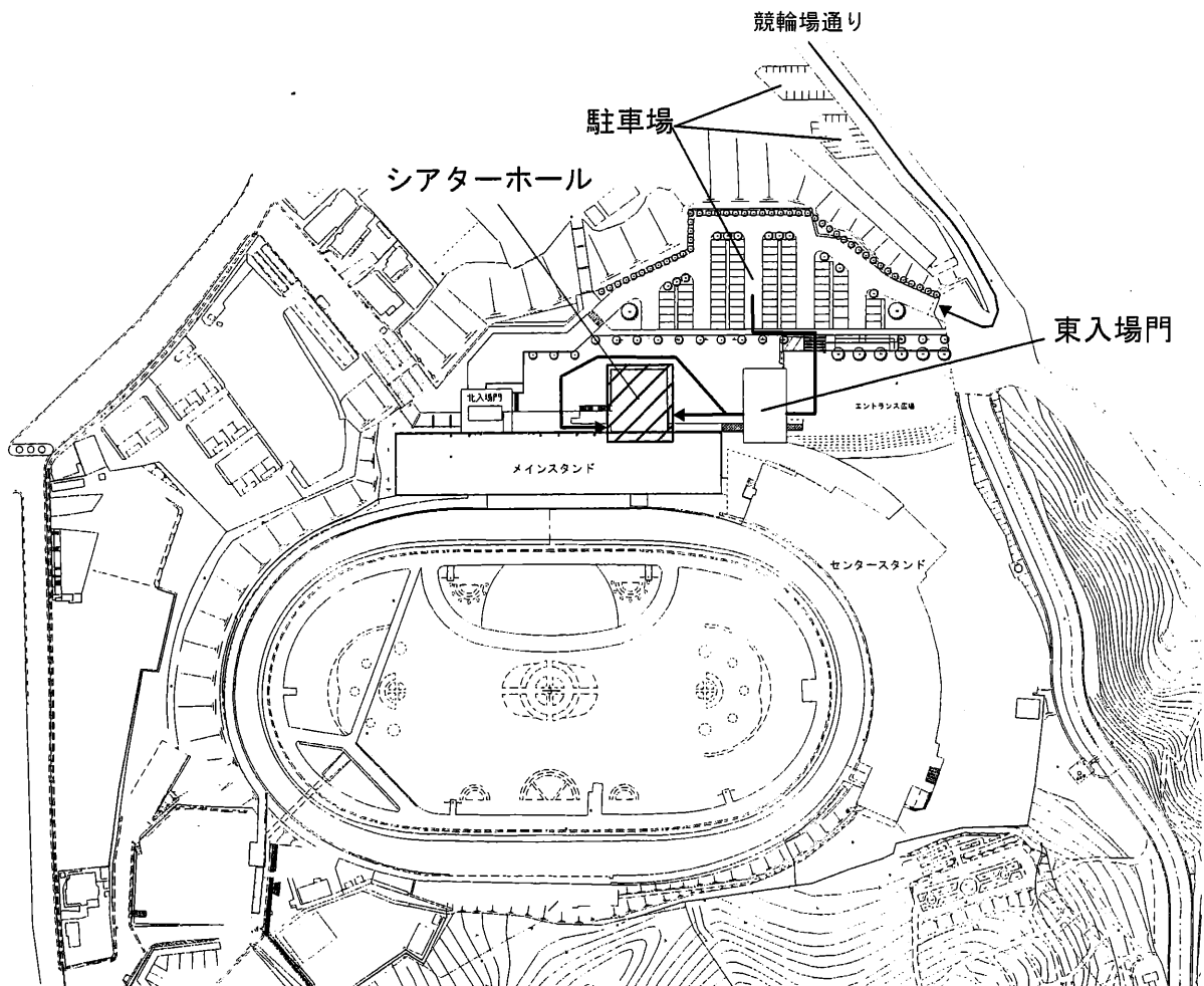
競輪場全体図
