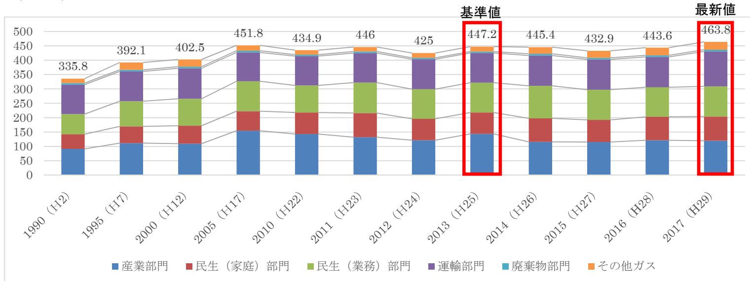
図1 宇都宮市の温室効果ガス排出量の推移
