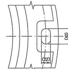
受枠7カ-穴詳細図
