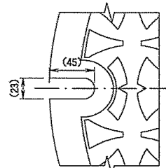
蓋開閉用穴詳細図
