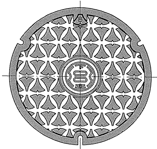
USM-A (T-14 汚水・合流用)
