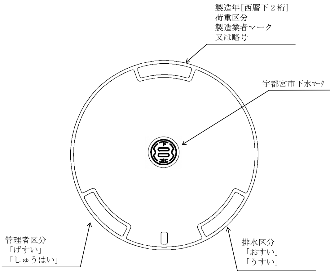
ふた表面図
