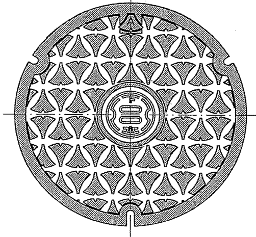
USM-A (T-14 汚水・合流用)
